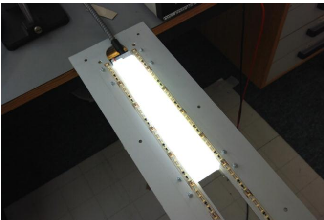
Figur 26 Foto af fiberlys koblet ud af lysblandingsklodsen. Hvide LEDer i hybridarmaturet er ikke tændt.
