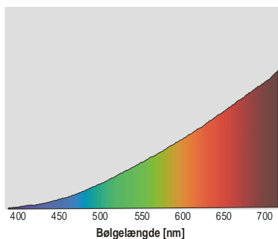
Figur 2. Bølgelængdespektrene for henholdsvis en glødepære (a) og et lysstofrør (b)
