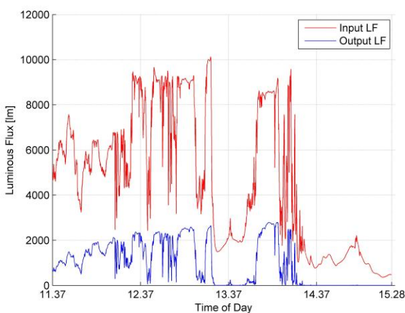
Figur 12 Grafen viser den målte lysstrøm der rammer linsearealet af SP3 systemet (rød linie) og den igennem fiberbunder transmitterede lysstrøm (blå linie), som funktion af tiden på dagen.
