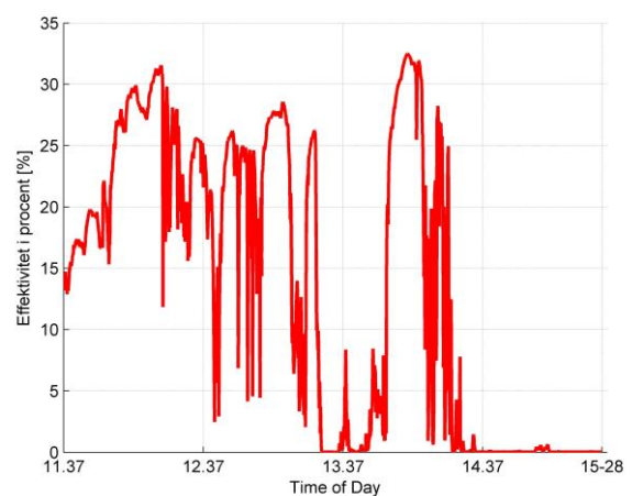
Figur 13 Målt effektivitet af SP3 system som funktion af tiden på dagen.
