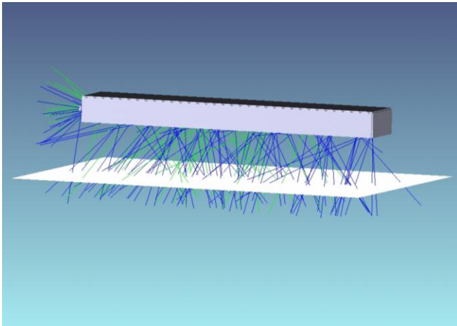
Figur 24 3D tegning af lysberegning på lysblandingsklods, der viser hvordan lysstråler fra fiberbundet (blå) og lysstråler fra LED (grøn) kobles ind i endebladen til venstre og kobles ud nedadrettet fra fra undersiden af klodsen.
