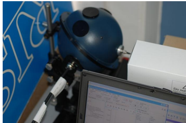
Figur 11 Integrerende kugle som opsamler alt lys transmitteret igennem et 20 m fiberbundet fra SP3 systemet og måles med et spektrometer
