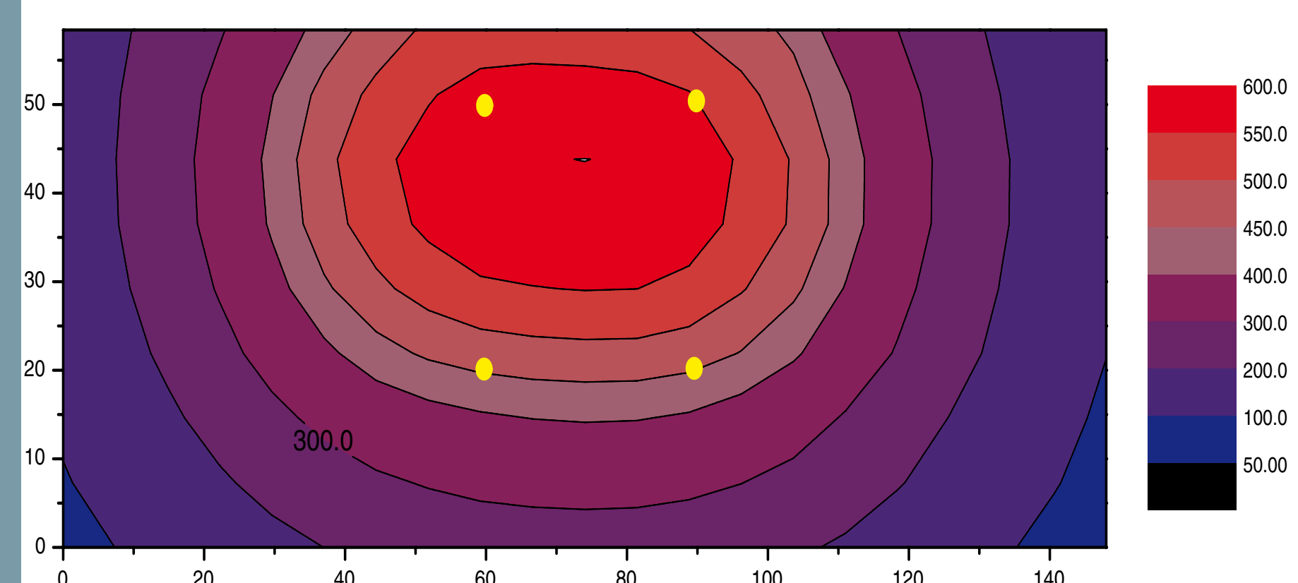
Målt lysfordeling i emhætte opstillingen med nye LED lyskilder med høj lyskvalitet, med et effektforbrug på 16.8 W. Øverst ses den målte belysningsstyrke [lux] på væggen under emhætten. Nederst ses den målte belysningsstyrke [lux] på arbejdsfladen under emhætten. De fire målepunkter markeret med gule cirkler svarer til centrum af fire kogezoneer. Grænsen for et belysningsstyrke niveau på 300 lux er markeret. Positionen langs akserne er angivet i cm. Det ses at LED lyskilderne giver en meget jævn lysfordeling over arbejdsfladen med belysningsstyrker på ca. 500 lux på alle fire kogezoneer.
