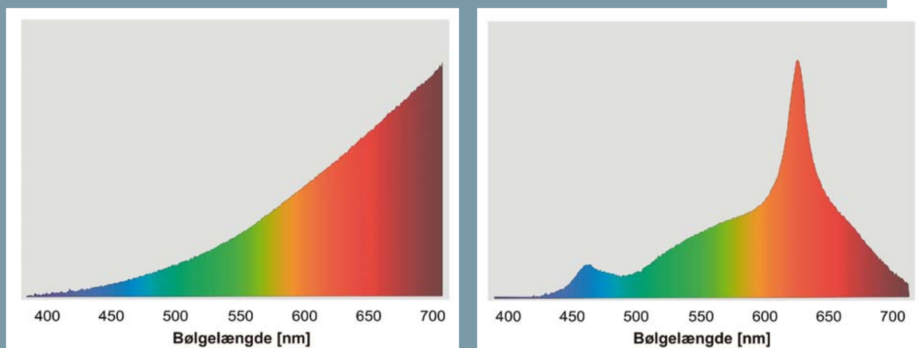
Til venstre: Målt farvesammensætning af lyset fra en 5 W pinol glødepære som traditionelt benyttes i skatkammerets montre. Til Højre: Den målte farvesammensætning af lyset fra den nye LED lyskilde til montrebelysning. Objekter set i lyset fra de to lyskilder vil se ens ud. Den største forskel ligger i at varmestrålingen (bølglængder over 700 nm) fra pinolglødepæren er kraftigt reduceret i LED lyskilden. Dette er en af grundene til den langt højere energieffektivitet af LED lyskilden.
