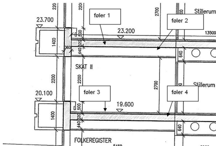
Figur 34. Tværsnit i bygning i plan 4 ved facade mod Skanderborgvej. Varmekapaciteten i etagedækket (320 mm huldæk+40 mm afretning) er ca. 150 Wh/m 2 /K.
