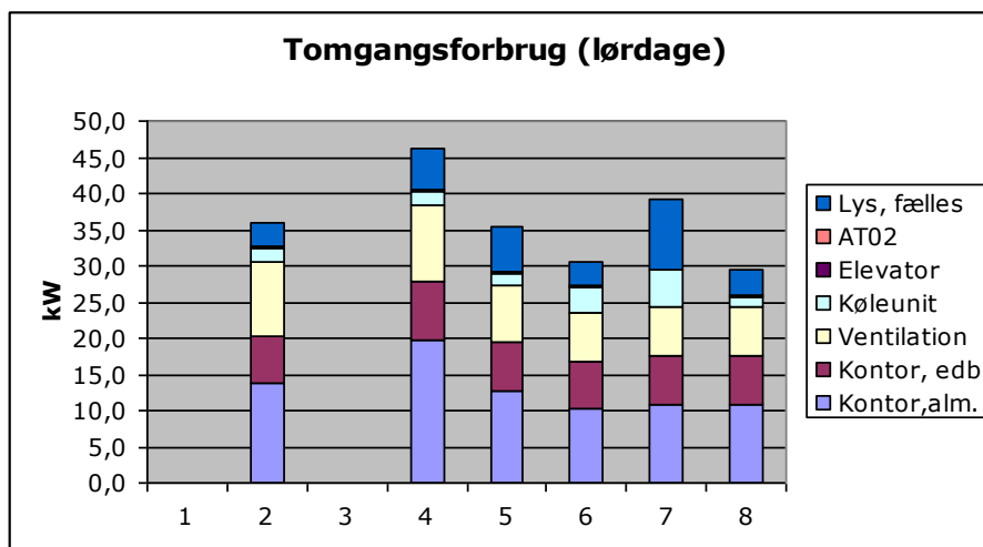
Figur 28. Tomgangseffekt middel ekskl. servere 2007-2008 på tilfældigt udvalgte lørdage. Søjle 2 er registreret i 2007 og de øvrige søjler stammer fra 2008.
