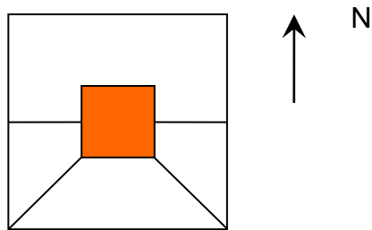
Figur 1. Punktformet bygning med syd-vest-, nord- og østvendte facader. Bygningens kerne, markeret med skravering, rummer servicefunktioner. Sidelængde af facade er 20 meter. Simulering af indeklimate og energiforbrug foretages på de tre vest-, syd- og østvendte zoner.
