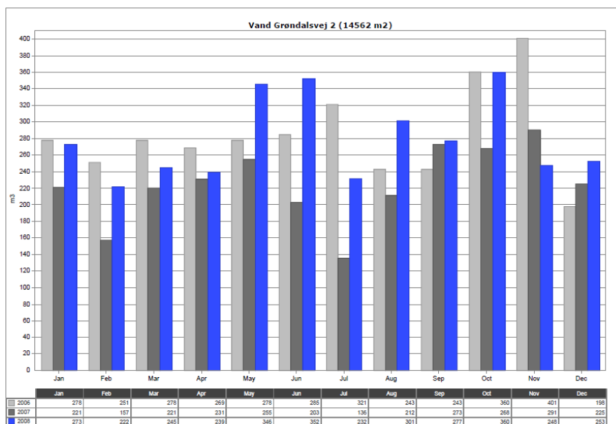
Figur 33. Diagrammet viser vandforbruget målt på hovedmåleren. Årsforbrug af vand fra den offentlige forsyning er ca. 3300 m 3 (pr. 1. september 2007-08). Varmt brugsvand udgør ca. 500 m 3 .
