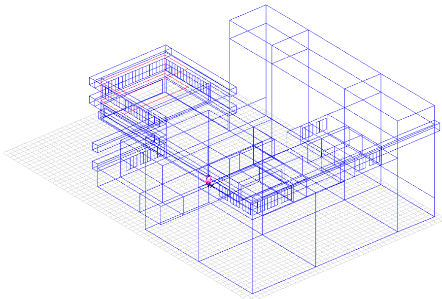
Figur 22. BSim-model af demonstrationsbyggeriet i Viby set fra syd. Den vestvendte fløj ovenpå kantinens, hvor specialrådgivningen for voksne med handicap skulle placeres, benævnt 'SR Ydre' i rapporten, er fremhævet med rødt.
