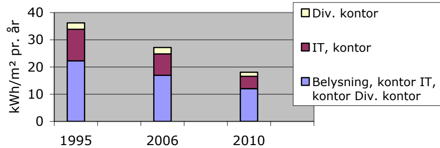
Figur 17. Ved anvendelse af ny teknik er det muligt at reducere varmebelastningen på grund af elforbrug i kontorområderne. Kølebehovet mindskes derved.
